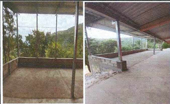
Foto 5: Area frontal donde se realizó Mejoramiento de muro de contención, mejoramiento de muro perimetral, Mejoramiento con estructura tipo portico y lámina troquelada calibre 26 y Mejoramiento de losa de piso.
